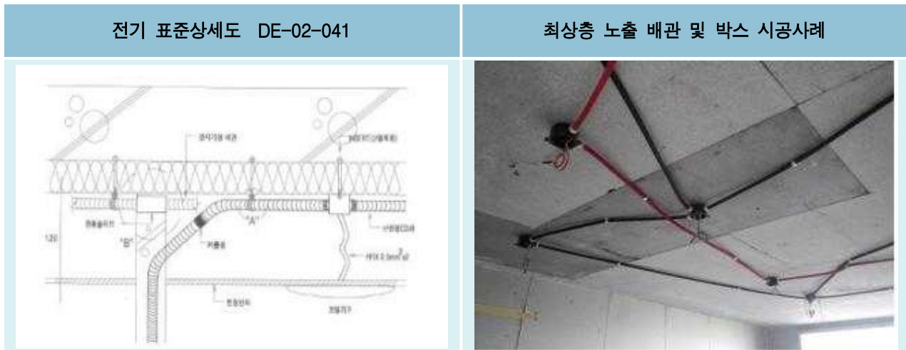
[그림 10] 최상층 배관 및 박스 공사
